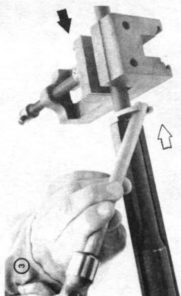
LOOSEN/TIGHTEN BAND
